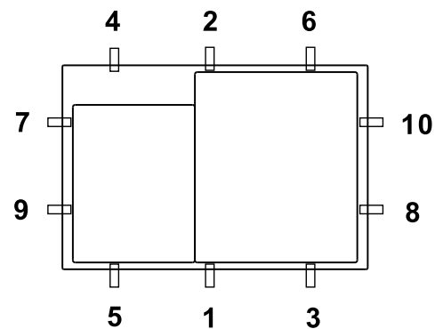
Séquence de serrage des clips
