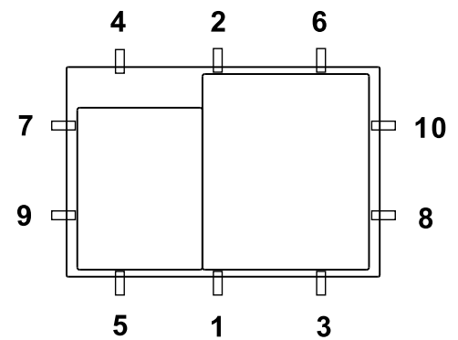
Secuencia de apriete de los clips
