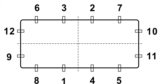
Secuencia de apriete de los clips
